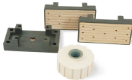
Įtarpai ir prispaudimo ratukai NK 016 95 x 48 x 25 mm ROL 013 Ø 62 x Ø 16 x 24 mm
