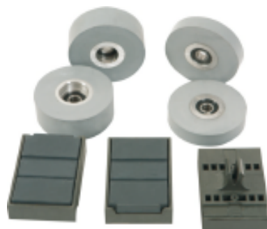
Įtarpai ir prispaudimo ratukai NK 006 71 x 48 x 18 mm ROL 003 Ø 65 x Ø 8 x 25 mm ROL 004 Ø 65 x Ø 8 x 14 mm
