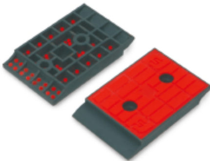
Įtarpai NKD 009 117 x 75 x 16,5 mm
