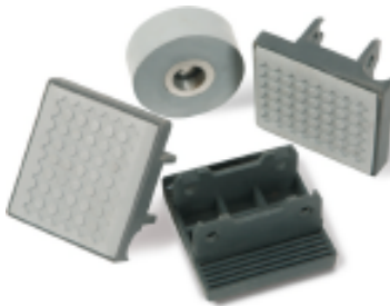
Įtarpai ir prispaudimo ratukai NK 015 79 x 72 x 18 mm ROL 012 Ø 65 x Ø 8 x 30 mm
