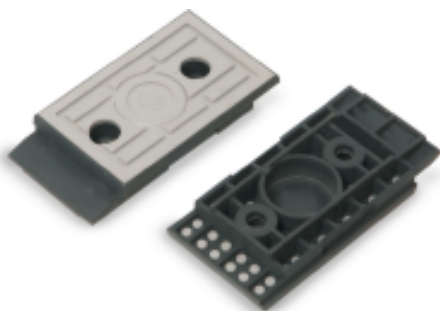
Įtarpai NKD 011 116 x 58 x 18 mm
