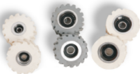
Prispaudimo ratukai ROL 017 \emptyset 65 x \emptyset 8 x 28 mm ROL 018 \emptyset 65 x \emptyset 8 x 14 mm ROL 019 \emptyset 65 x \emptyset 12 x 28 mm ROL 020 \emptyset 65 x \emptyset 12 x 14 mm
