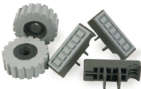
Įtarpai ir prispaudimo ratukai NK 005 80 x 30 x 18 mm ROL 002 Ø 70 x Ø 20 x 25 mm
